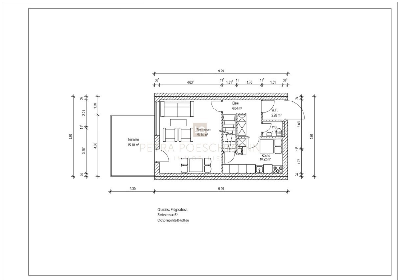
GR Erdgeschoss
